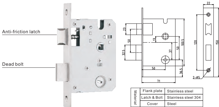
Mortise 5050
