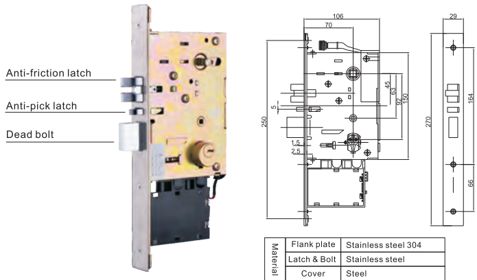
Mortise ANSI-L
