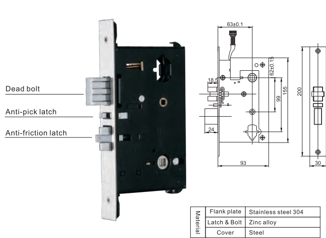
Mortise ANSI 2#
